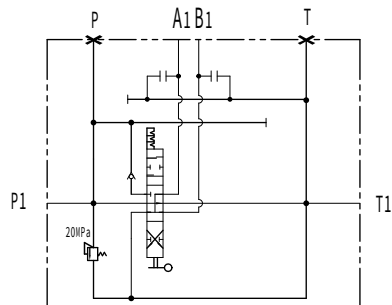
液压原理图
